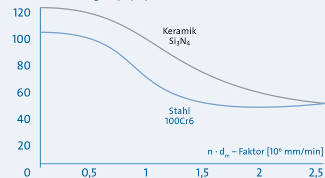
Radiale Steifigkeit [N/μm]
