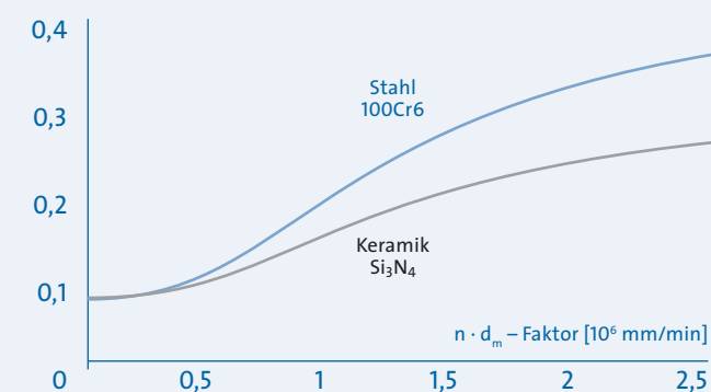
Bohr-/Roll-Verhältnis
